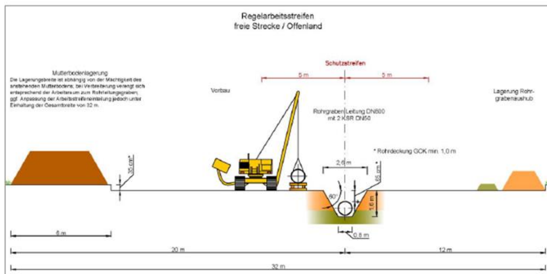
Abbildung 3: Regelarbeitsstreifen in freier Strecke
